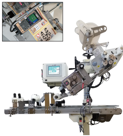
上貼シール機 EG-8000II
